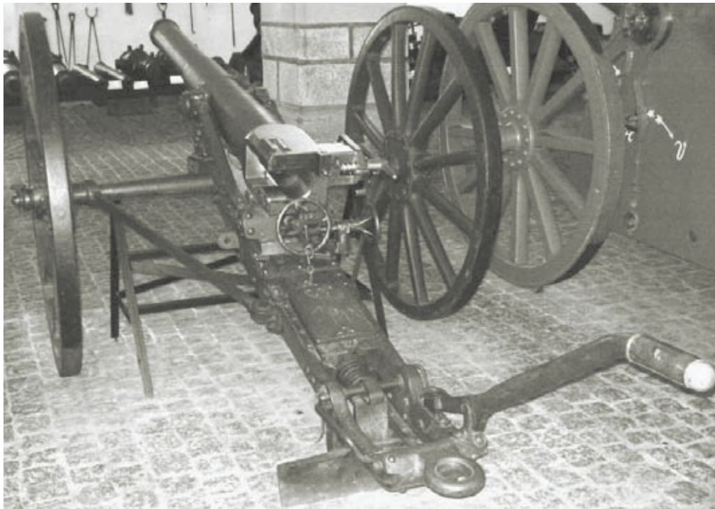
Den Schouboe'ske nødløsning efter tabet af de fire feltkanoner: 75 mm stålkanon L/28 M1894. (Forfatterens foto fra Statens Forsvarshistoriske Museum)
